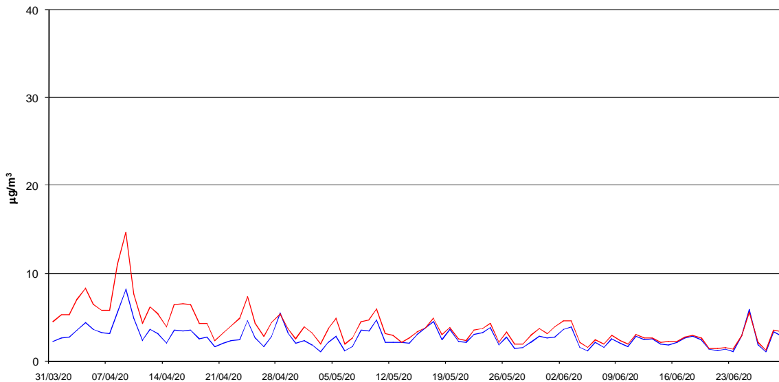
Чађ - аутоматски-селективна двоканална анализа дневне концентрације ВС&УVкомпоненти мерно место Стрелиште II квартал 2020. године
