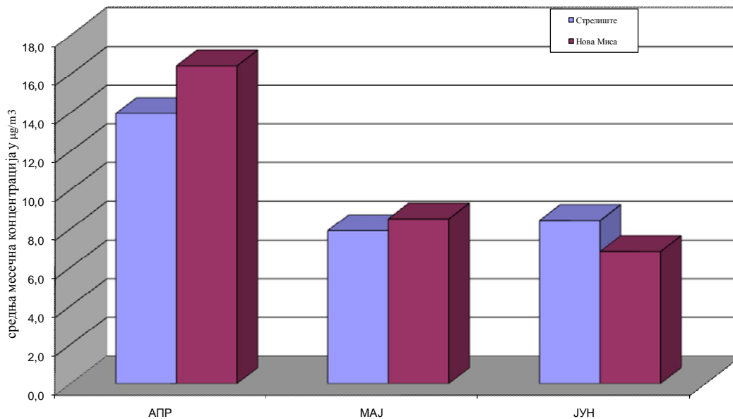
ЧАЂ У ВАЗДУХУ АМБИЈЕНТА Мерна места: Стрелиште и Нова Миса Панчево, IV-VI 2020. Дистрибуција просечних месечних концентрација чађи у \mu\text{g}/\text{m}^3
