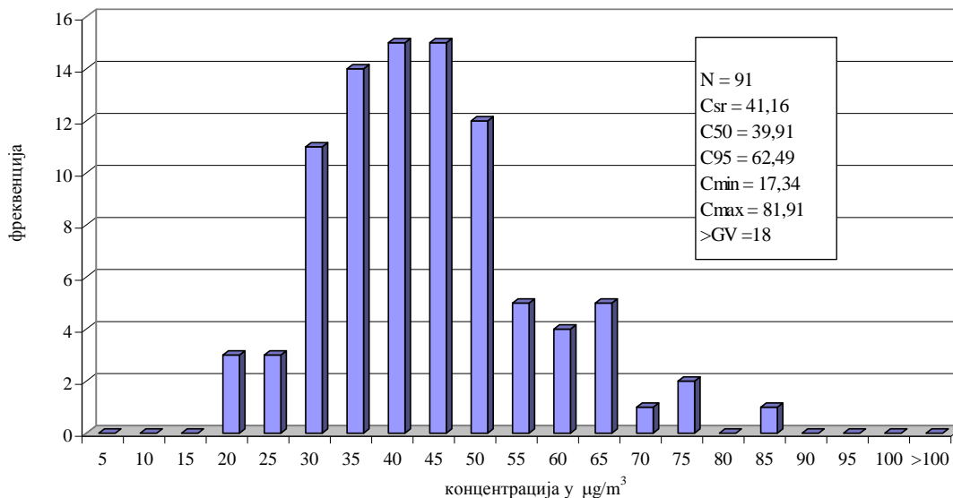
PM10 у ваздуху амбијента Мерно место: Панчево, Народна башта II квартал 2017.године Дистрибуција релативних фреквенција 24h концентрација аутоматски мониторинг
