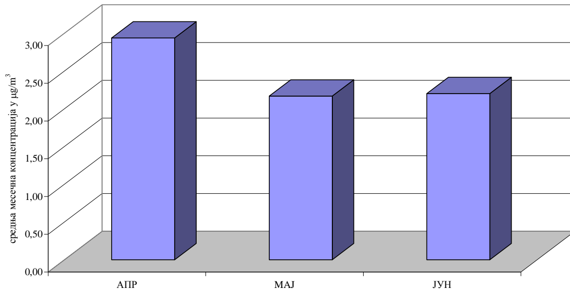
Толуен у ваздуху амбијента Мерно место: Панчево, Народна башта II квартал 2017.године Сезонска дистрибуција средњих месечних концентрација ( \mu\text{g}/\text{m}^3 ) аутоматски мониторинг
