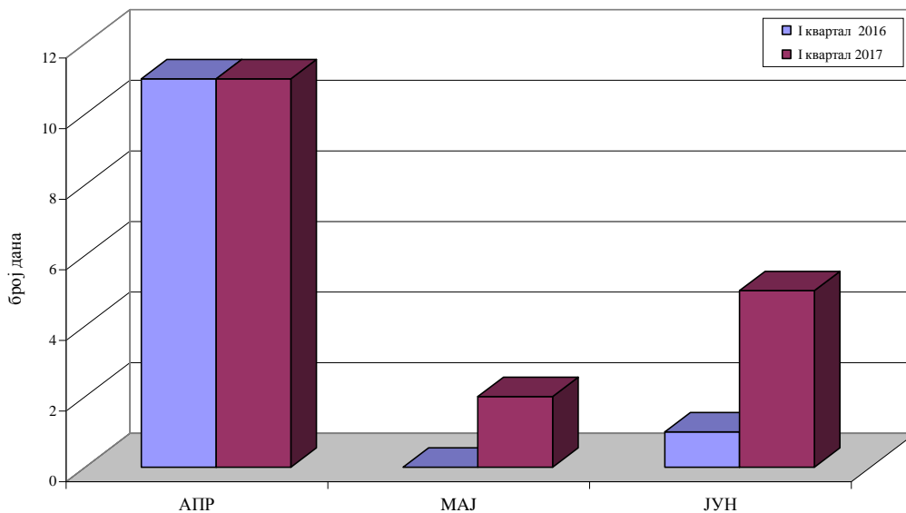
PM10 У ВАЗДУХУ АМБИЈЕНТА Мерно место: Панчево, Народна башта Упоредни приказ броја дана са концентрацијама изнад GV II квартал 2016.-II квартал 2017.
