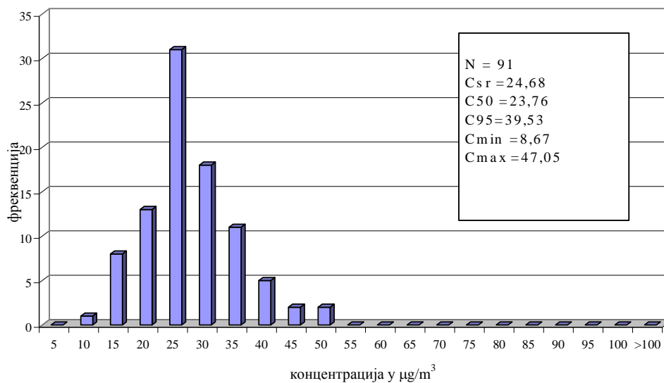
PM2,5 у ваздуху амбијента Мерно место: Панчево, Народна башта II квартал 2017.године Дистрибуција релативних фреквенција 24h концентрација аутоматски мониторинг
