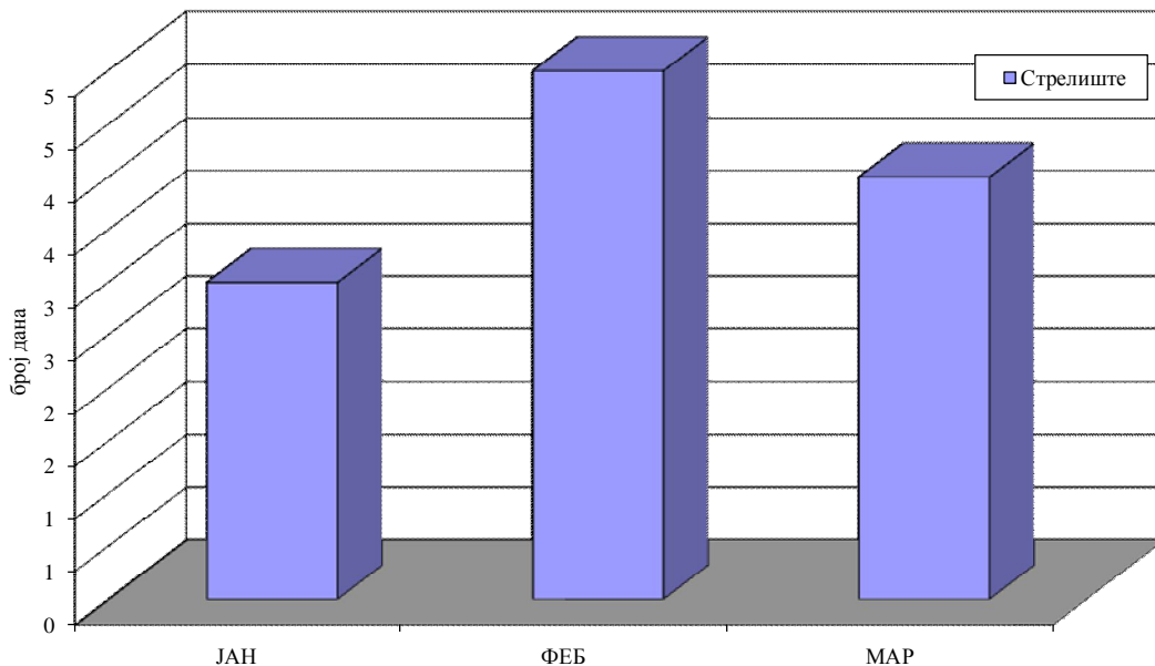
PM10 У ВАЗДУХУ АМБИЈЕНТА Мерно место: Панчево, Стрелиште I квартал 2018.године Број дана са концентрацијама PM10 изнад GV
