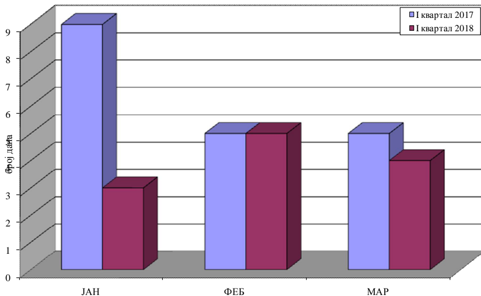
PM10 У ВАЗДУХУ АМБИЈЕНТА Мерно место: Панчево, Стрелиште упоредни приказ броја дана са концентрацијама изнад GV I квартал 2017. - I квартал 2018.
