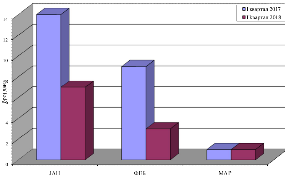
ЧАЂ У ВАЗДУХУ АМБИЈЕНТА Мерно место: Панчево, Нова Миса Упоредни приказ броја дана са концентрацијама изнад GV I квартал 2017. - I квартал 2018.
