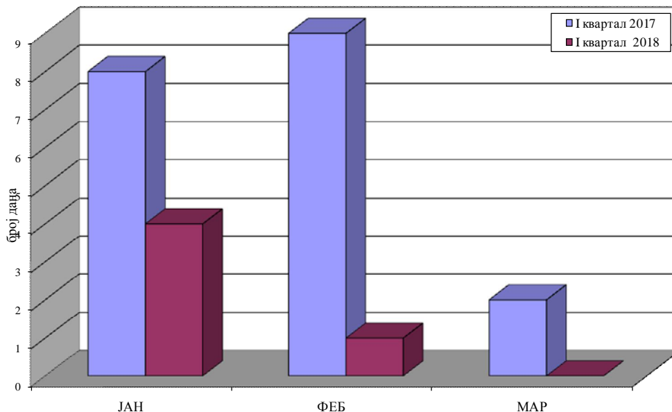
ЧАЂ У ВАЗДУХУ АМБИЈЕНТА Мерно место: Панчево, Стрелиште Упоредни приказ броја дана са концентрацијама изнад GV I квартал 2017. - I квартал 2018.
