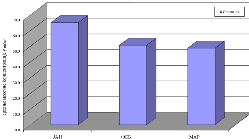
PM 10 У ВАЗДУХУ АМБИЈЕНТА Мерно место: Панчево, Стрелиште I квартал 2018.године Дистрибуција средњих месечних концентрација у \mu\text{g}/\text{m}^3
