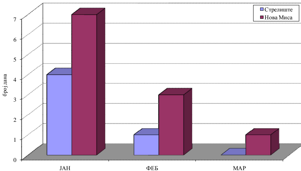
ЧАЂ У ВАЗДУХУ АМБИЈЕНТА Мерно место: Панчево, Стрелиште и Нова Миса I квартал 2018. године Број дана са концентрацијама изнад \text{GV}
