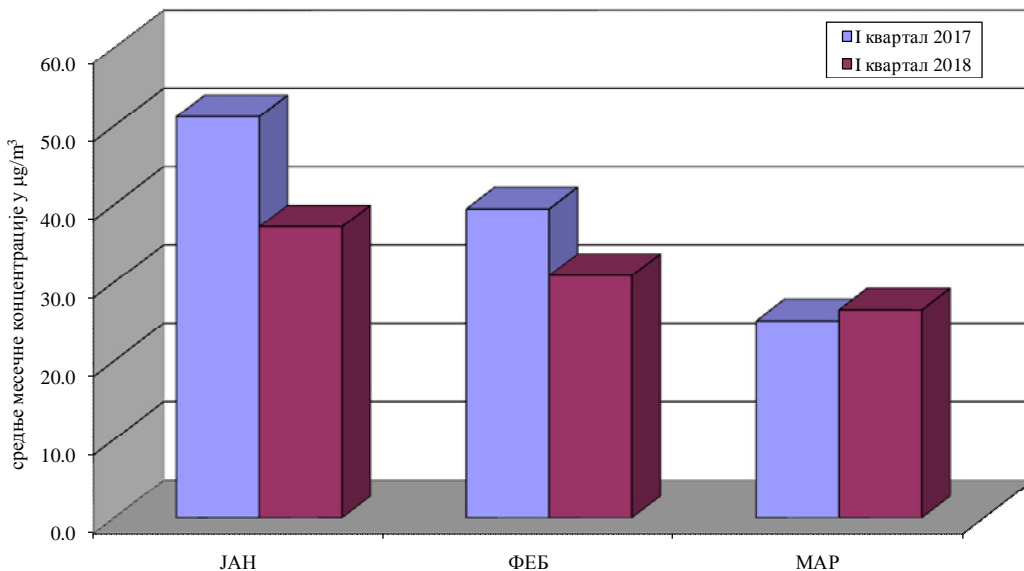
ЧАЂ У ВАЗДУХУ АМБИЈЕНТА Мерно место: Панчево, Нова Миса Упоредни приказ средњих месечних концентрација у \mu\text{g}/\text{m}^3 I квартал 2017. - I квартал 2018.
