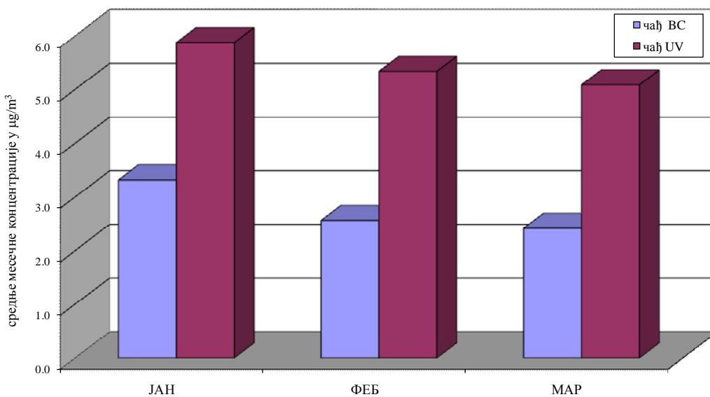
ЧАЂ У ВАЗДУХУ АМБИЈЕНТА Мерно место: Панчево, Стрелиште I квартал 2018.године Селективна двоканална анализа чађи (BC&UV) Приказ средњих месечних концентрација чађи у \mu\text{g}/\text{m}^3
