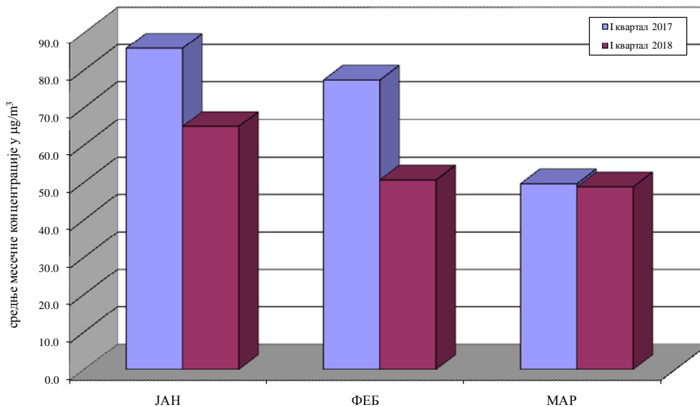
PM 10 У ВАЗДУХУ АМБИЈЕНТА Мерно место: Панчево, Стрелиште упоредни приказ средњих месечних концентрација PM 10 у \mu\text{g}/\text{m}^3 I квартал 2017. - I квартал 2018.
