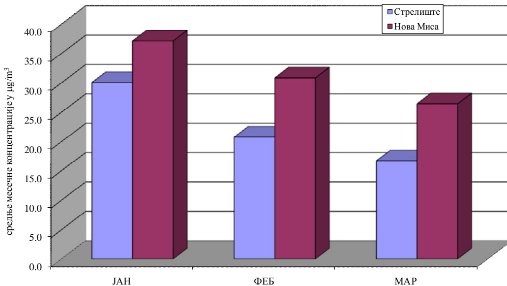
ЧАЂ У ВАЗДУХУ АМБИЈЕНТА Мерно место: Панчево, Стрелиште и Нова Миса I квартал 2018.године Дистрибуција средњих месечних концентрација чађи у \mu\text{g}/\text{m}^3
